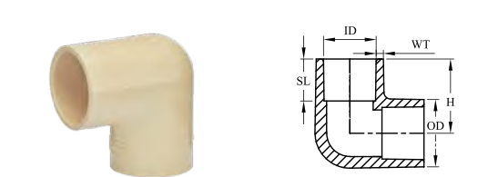
ELBOW 90° (SCH 80)
