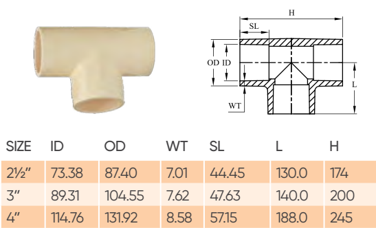
TEE 90° (SCH 40)
